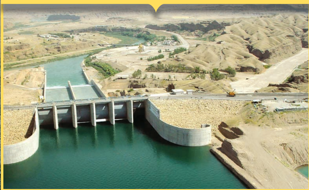
سد کرخه با ظرفیت ۵/۵ میلیارد مترمکعب
