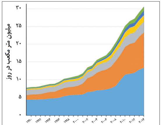
شکل ۳- ظرفیت تولید آب شیرین با استفاده از نیروگاه های برق در همسایه های جنوبی کشور
